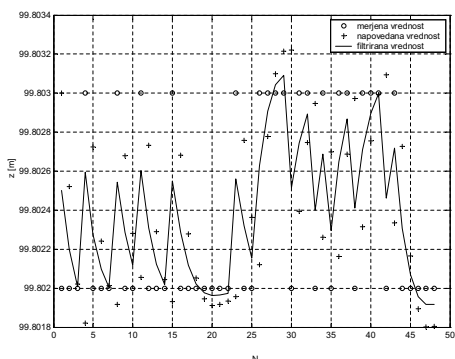
Slika 4: Merjene, napovedane in filtrirane vrednosti komponent položaja reflektorja za q=0.00001
