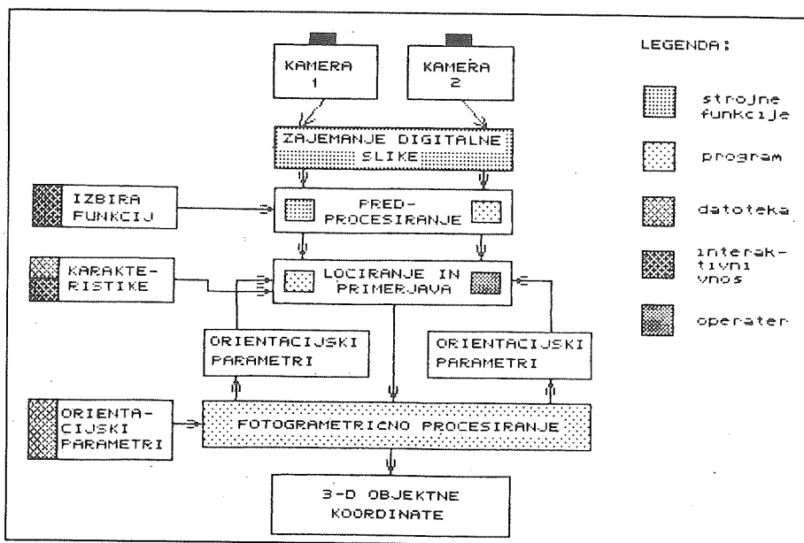
Blok diagram osnovnih operacij za izvedenost digitalnih posnetkov Slika 4.5
