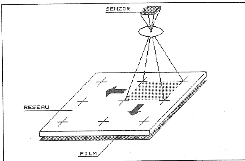
Princip "reseau-scanninga", kot je uporabljen v reseau - skanerju RS1 firme Rollei Slika 4.1
