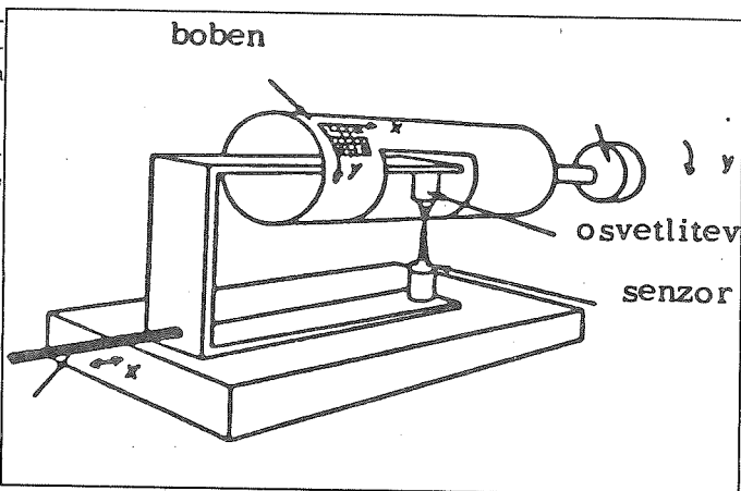
Scanner z vrtečim valjem Slika 2
