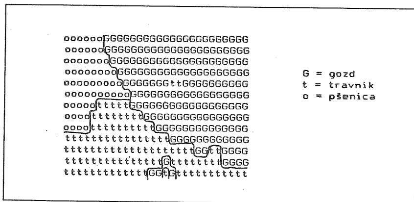
Slika 5b: kartografski izpis pixlov, razvrščenih v 3 razrede izrabe tal
