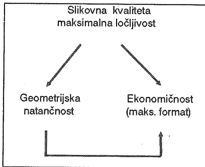
Slika 1: Trikotnik optimiranja
