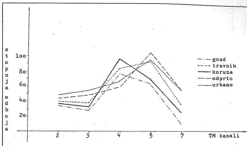
Slika 6: povprečne vrednosti odboja vadbenih vzorcev petih razredov izrabe tal območja občine Ajdovščina, skanirano s TM-Landsat satelitom 2.8.86
