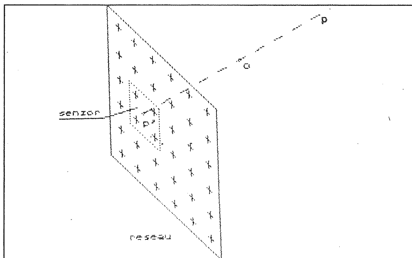
Princip "reseau-scanning" v fotogrametrični kameri
