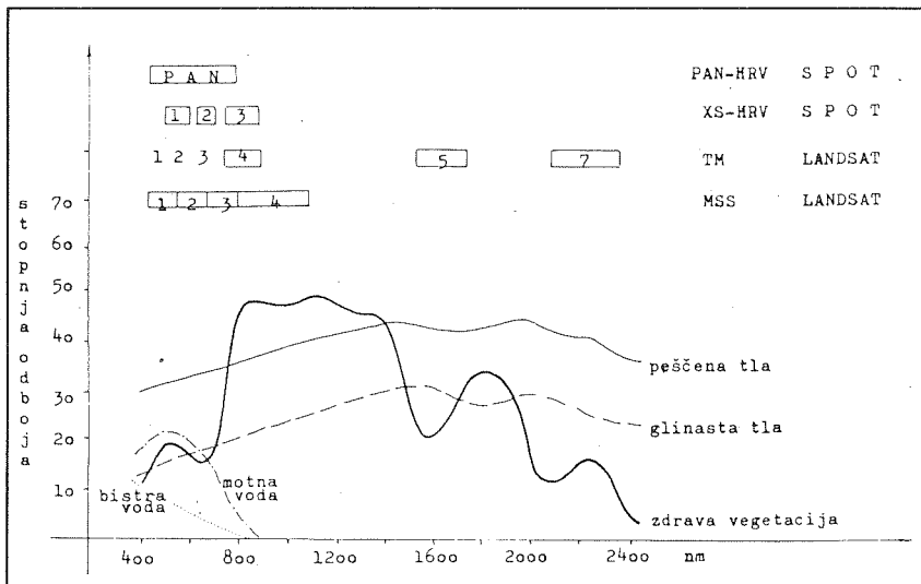
Slika 3: značilne spektralne krivulje odboja in vpijanje EMV nekaterih pojavov-predmetov na površini Zemlje ter občutljivost detektorjev na skanerjih satelitov
