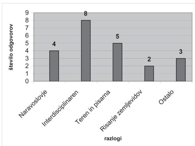
Graf 1: Razlogi odločitve za študij geodezije.
