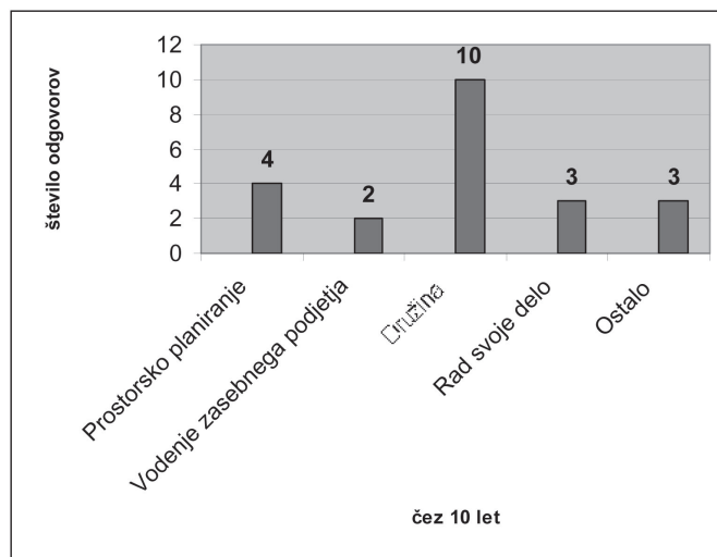
Graf 3: Videnje čez 10 let.
