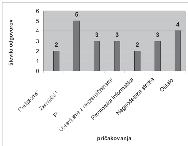
Graf 2: Želje po končanem študiju.
