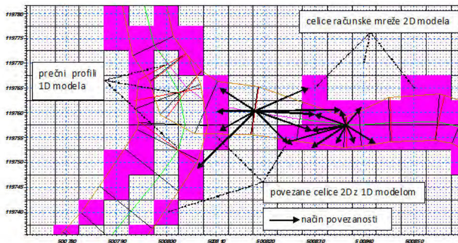
Slika 4: Izsek sestavljenega modela MIKE FLOOD, povezane celice 2D-komponente, prečni profili 1D-komponente, način povezovanja z lateralnimi povezavami.
