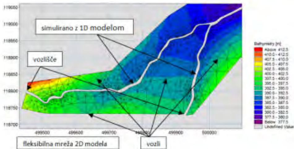
Slika 3: Fleksibilna (trikotna) računsko mreža 2D-modela
